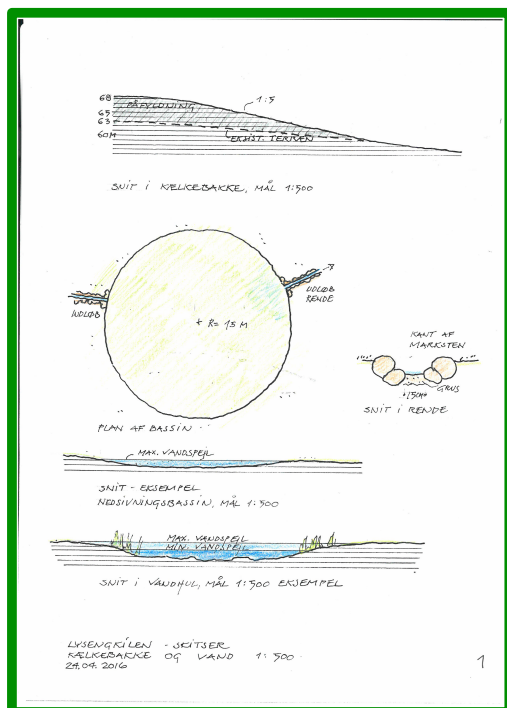
Skitse af kælkebakke samt plan og og snit i et nedsivningsbassin
