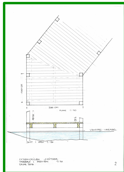
Skitse af træbro
